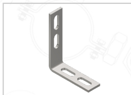
ESCUADRA REFUERZO 27 - 90°
